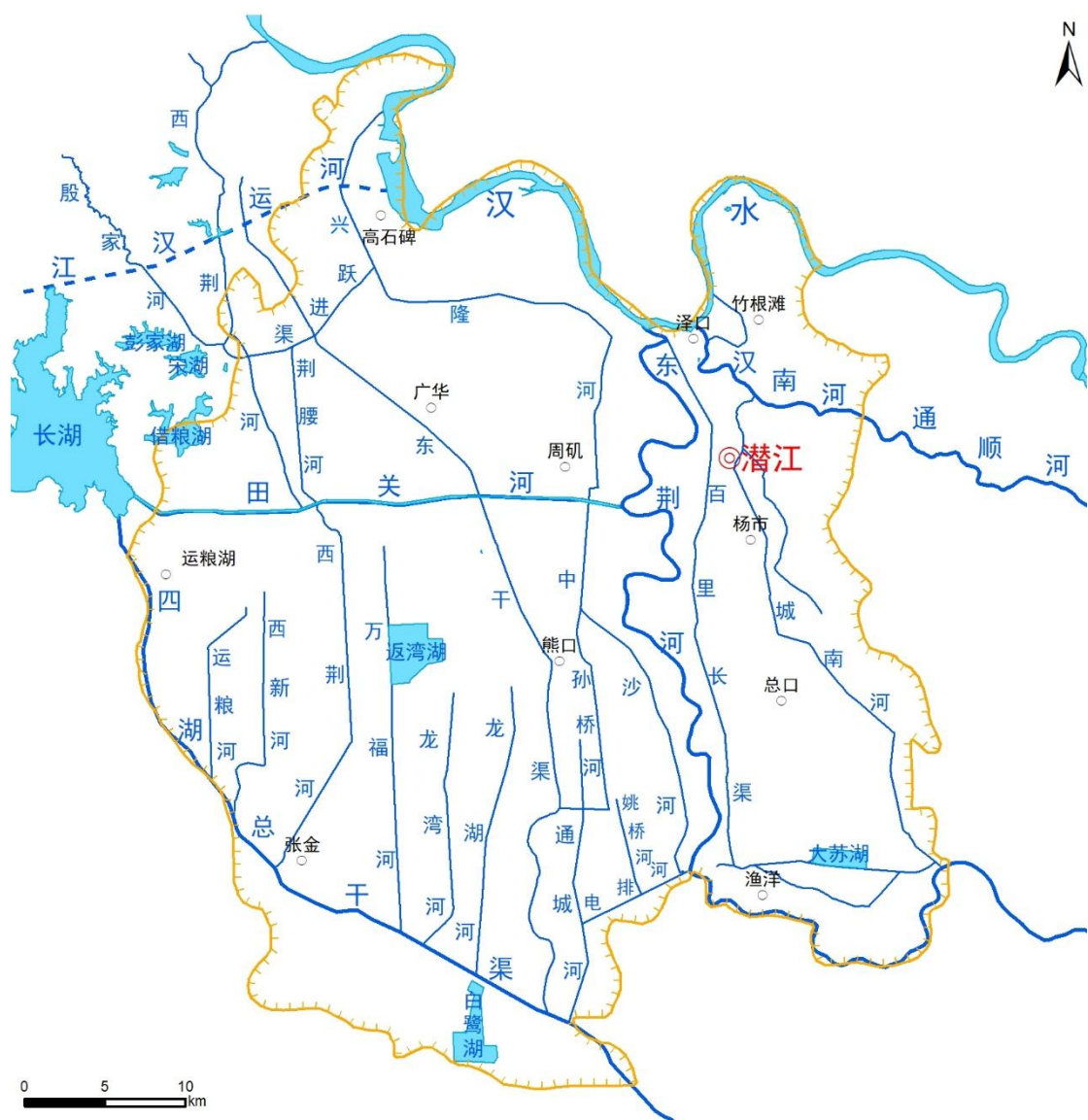
图 2.3-2 区域水系图
